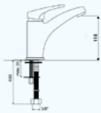
модел RI122 СМЕСИТЕЛ СТОЯЩ ЗА КЕРАМИЧНА МИВКА
