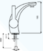
модел LX102 100% МЕСИНГ
