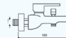
модел LX101 100% МЕСИНГ
