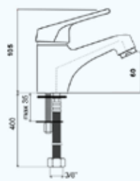
модел DA102 100% МЕСИНГ
